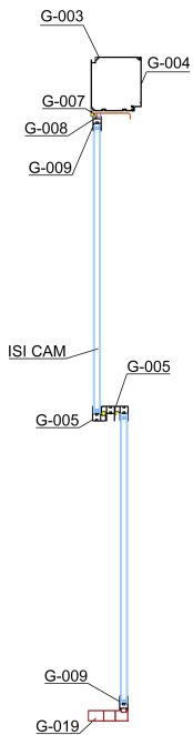
A-A KESİTİ
