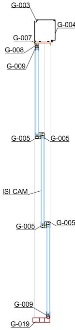
A-A KESİTİ
