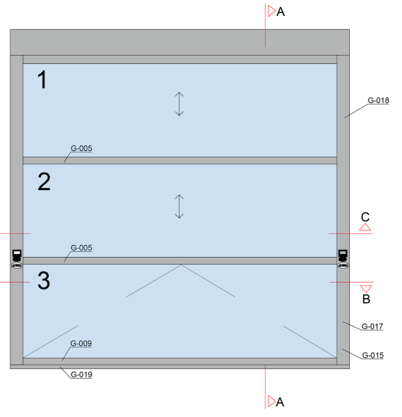
ÖN GÖRÜNÜŞ
