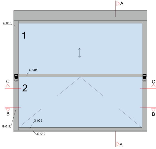
ÖN GÖRÜNÜŞ
